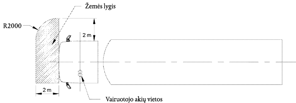
11 paveikslas. VI klasės priekinio veidrodžio matymo laukas
