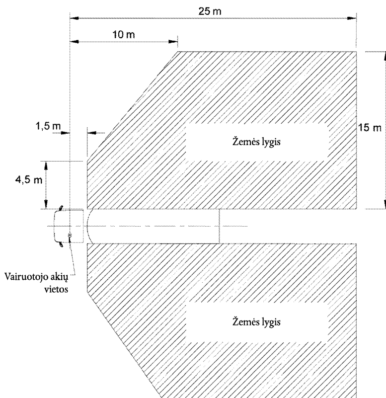
9 paveikslas. IV klasės plačiakampių veidrodžių matymo laukas
