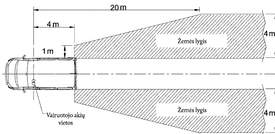
8 paveikslas. III klasės veidrodžių matymo laukas
