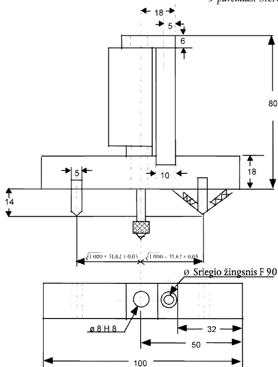
3 paveiklas. Sferometras
