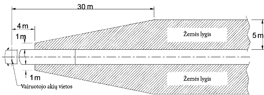
7 paveikslas. II klasės veidrodžių matymo laukas
