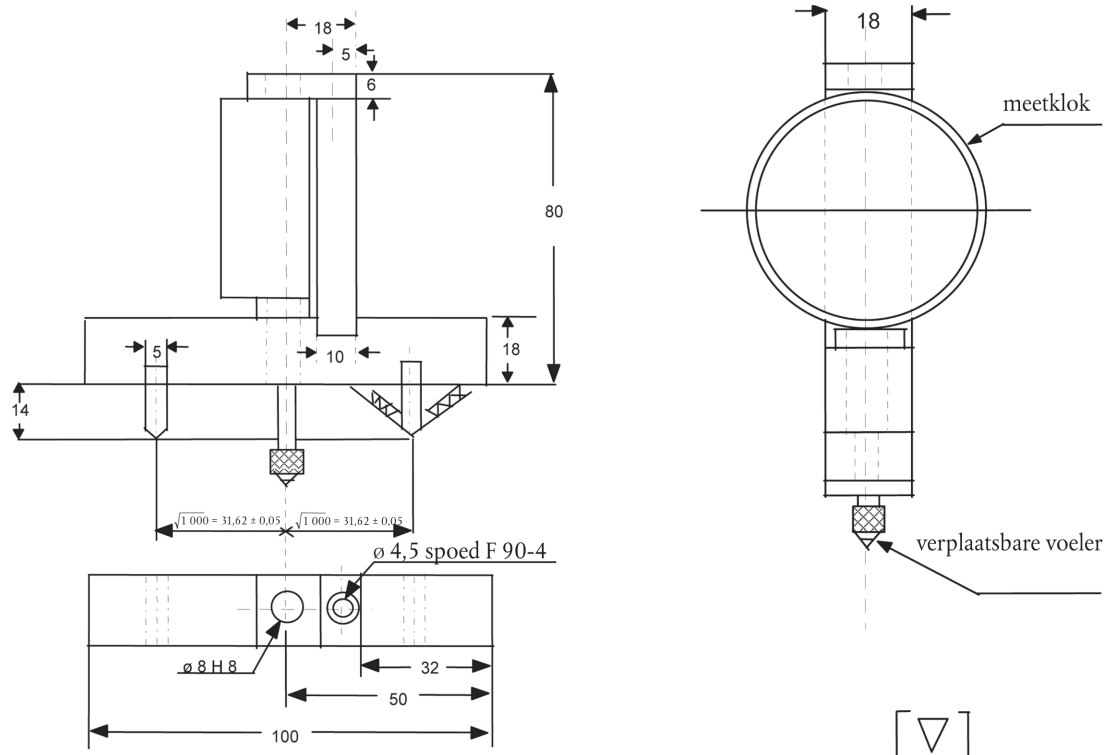
Figuur 3: Sferometer
