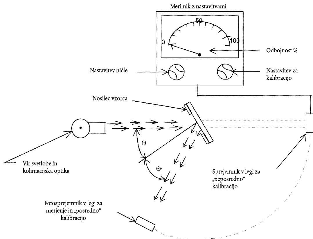
Slika 4: Osnovna shema aparata za merjenje odbojnosti po obeh postopkih kalibracije
