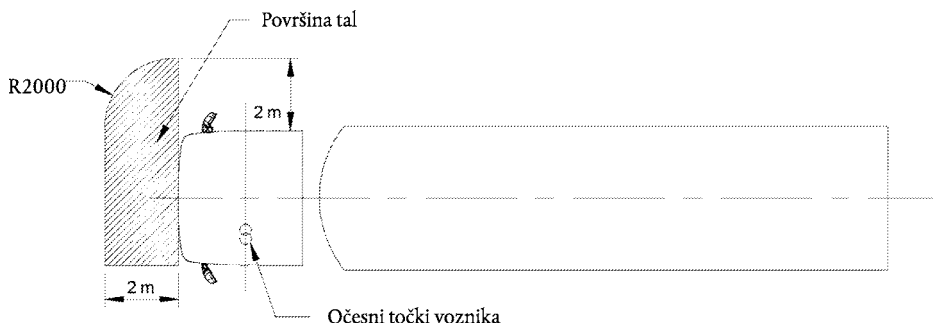
Slika 11: Vidno polje prednjega ogledala razreda VI
