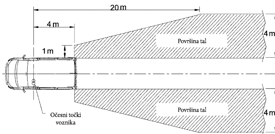
Slika 8: Vidno polje ogledal razreda III
