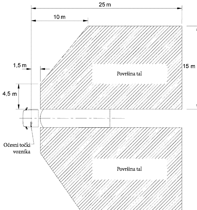
Slika 9: Vidno polje širokokotnih ogledal razreda IV
